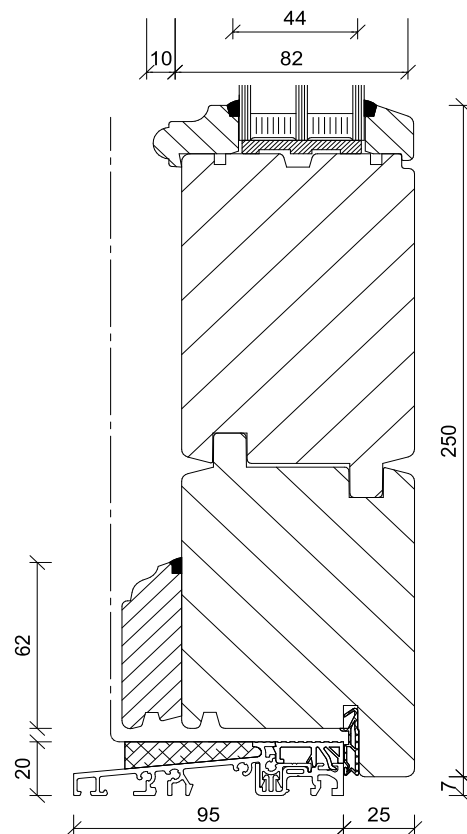
Schnitt: Ausführung profiliert
