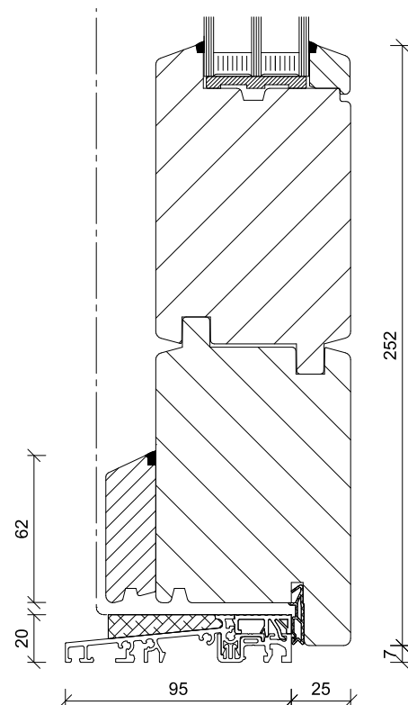
Schnitt: Ausführung gerade
